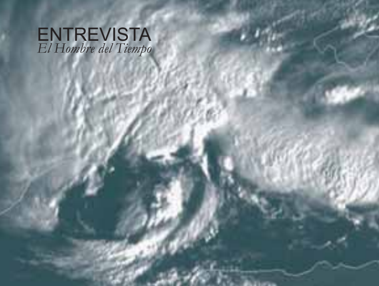
Formación de Gota Fría
